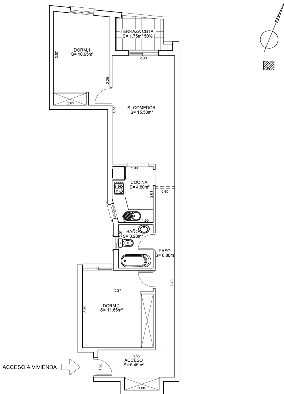
PLANTA PISO
